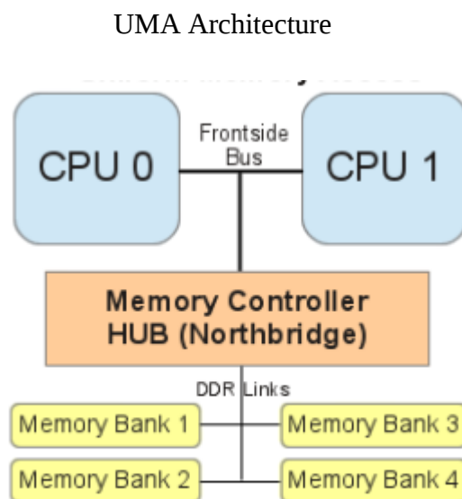
Figure 2-1 UMA Architecture
